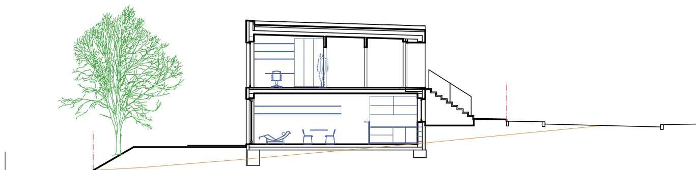
řez příčný
