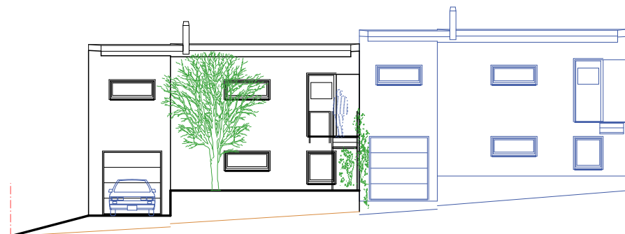
pohled uliční
