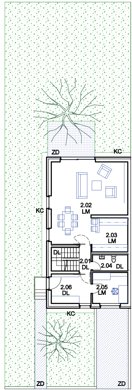
půdorys 2. nadzemního podlaží
