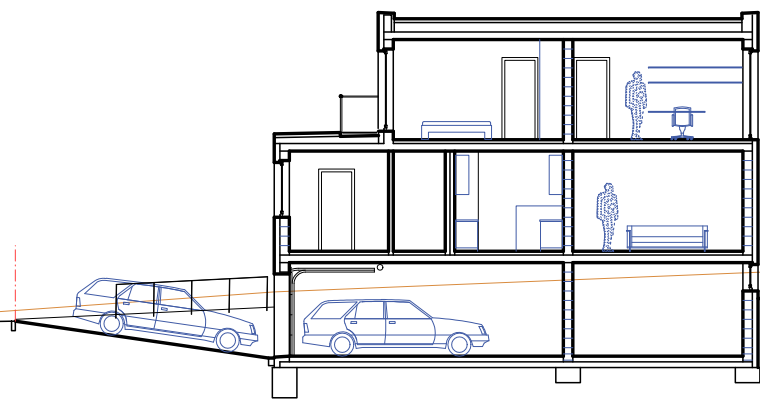
286.000 řez příčný
