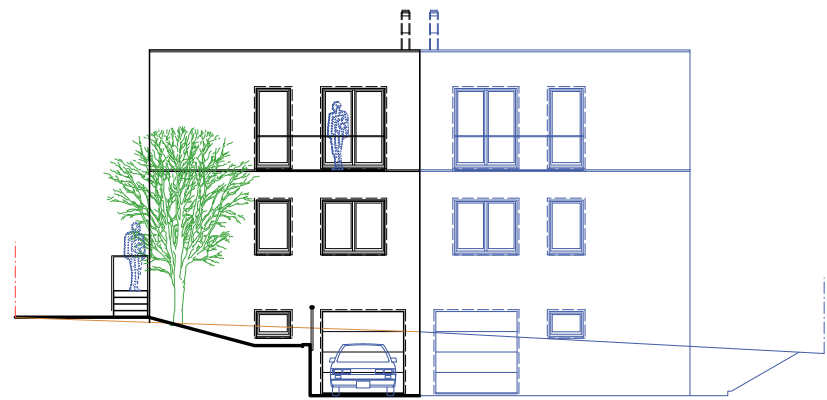
286.000 pohled zahradní
