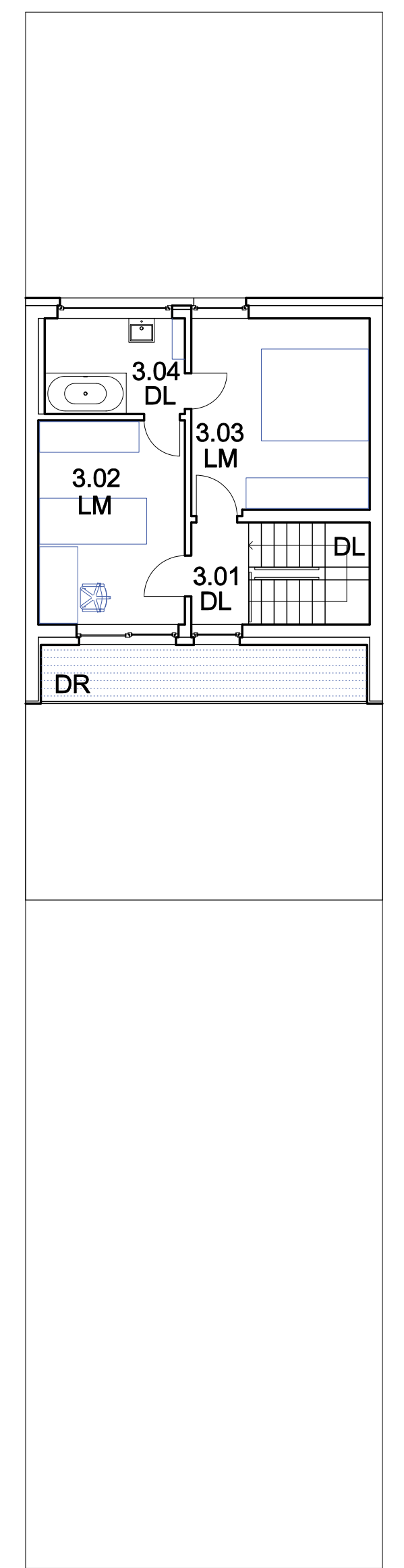
půdorys 2. nadz. podl.
