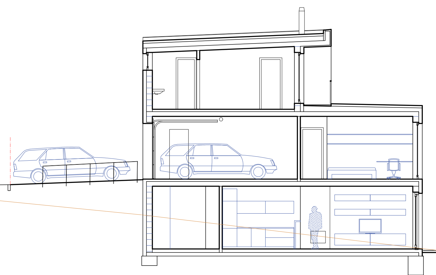
řez příčný
