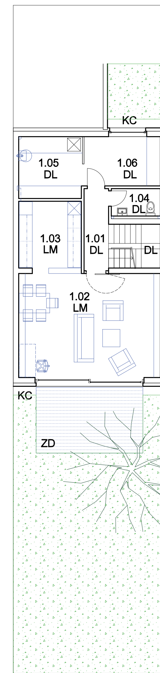
půdorys 1. nadz. podl.
